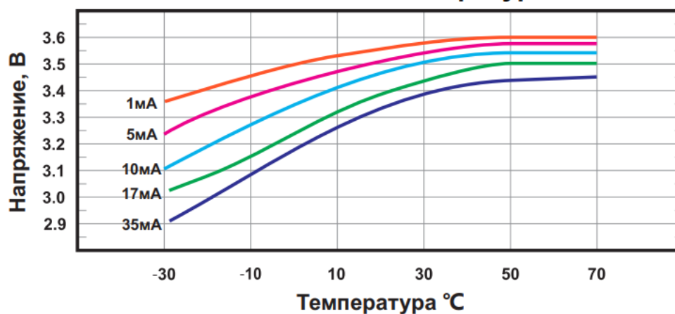
Зависимость напряжения от силы тока и температуры
